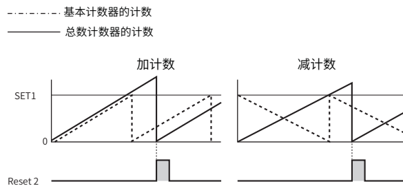
方式1/2/3 OUT2无/计数继续
