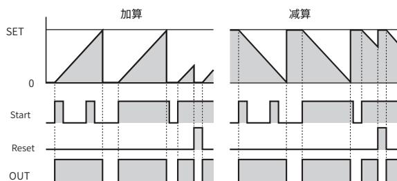
方式C 单脉冲
