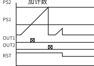
方式6 OUT1:脉冲输出 OUT2:脉冲输出, 计数复位
