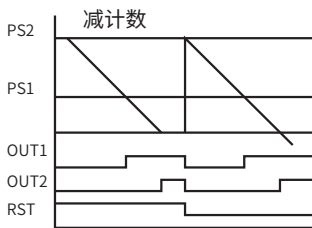
方式2 OUT1:输出保持 OUT2:脉冲输出, 计数复位
