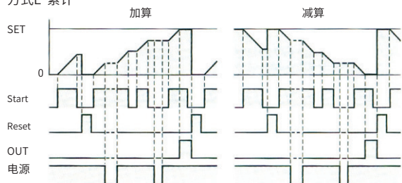
方式E 累计
