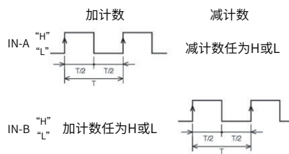
加减分别输入/正逻辑输入
