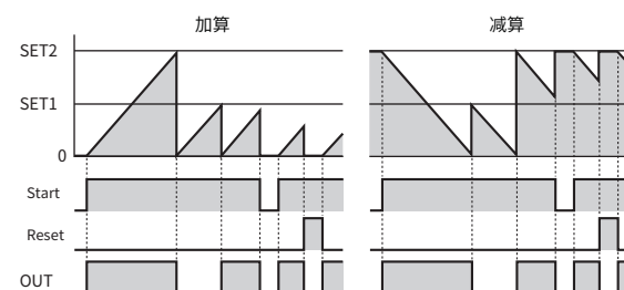
方式D 闪烁、触发
