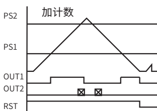
方式3 OUT1:输出保持 OUT2:脉冲输出, 计数继续
