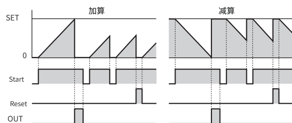
方式A ON输出
