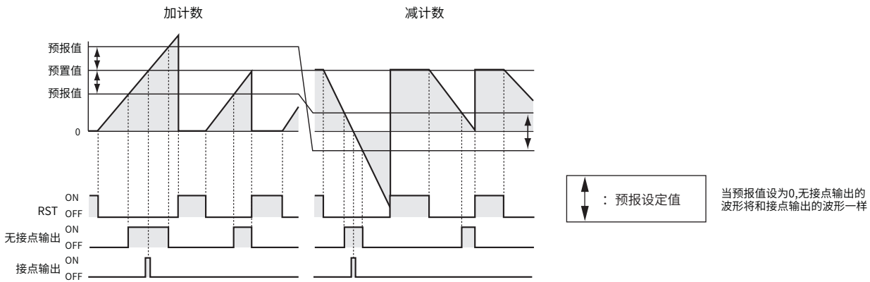
一致输出,计数继续
