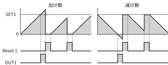
方式2/5/8 OUT1脉冲输出/计数复位
