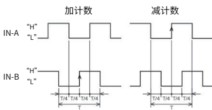
两相输入方式
