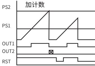
方式2 OUT1:输出保持 OUT2:脉冲输出, 计数复位
