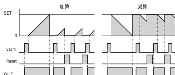
方式B OFF输出
