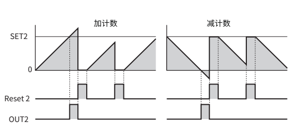
方式7/8/9 OUT2脉冲输出/计数继续
