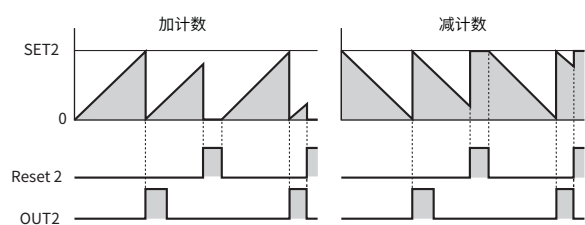
方式4/5/6 OUT2脉冲输出/计数复位
