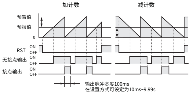
脉冲输出,计数复位
