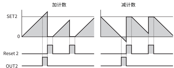
方式1/2/3 OUT2输出保持/计数继续
