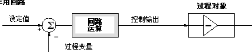
反作用回路
